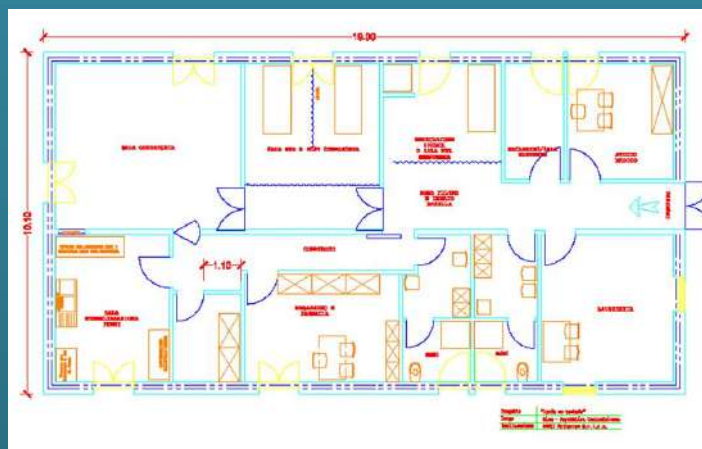
2) Planimetria/progetto del nuovo blocco operatorio
